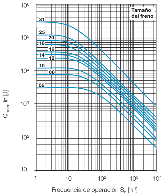
Figura 6 – Curva de disipación de calor (Q) por arranques por hora.
